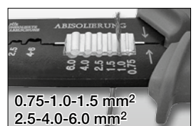
0.75-1.0-1.5 mm 2 2.5-4.0-6.0 mm 2 Abisolierzange für Kabel Dénudage de câbles Spellafili per cavi
